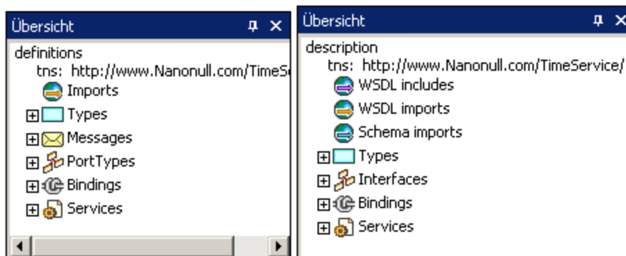
Eingabehilfe "Übersicht" in WSDL 1.1 (links) und WSDL 2.0 (rechts)
